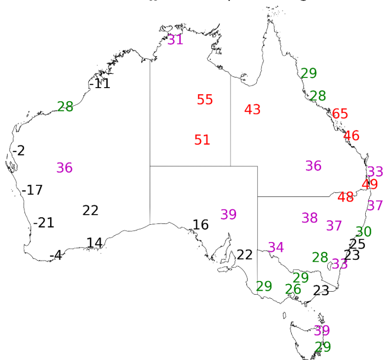
SON FFDI90-JJA ENSO partial lag=1
