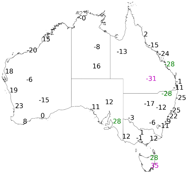
DJF FFDI90-JJA SAM partial lag=2
