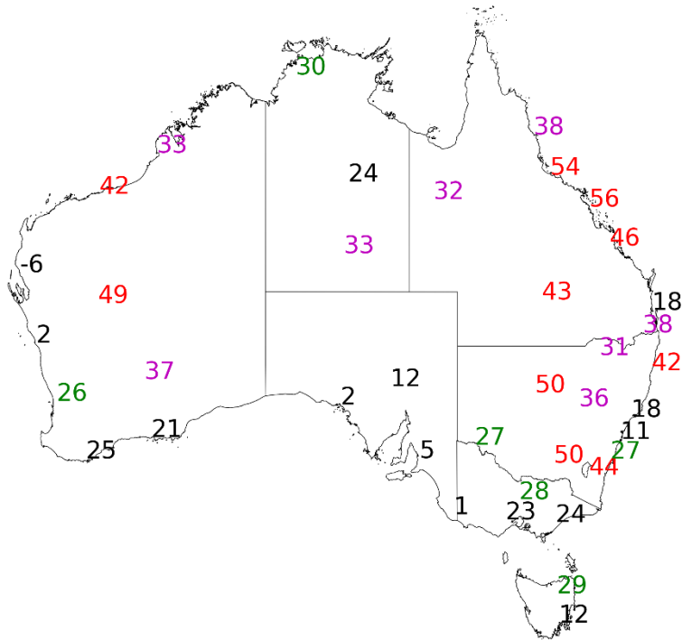
DJF FFDI90-JJA ENSO partial lag=2
