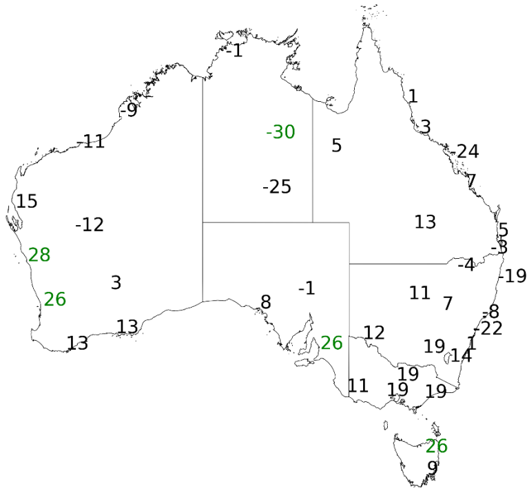
SON FFDI90-JJA SAM partial lag=1
