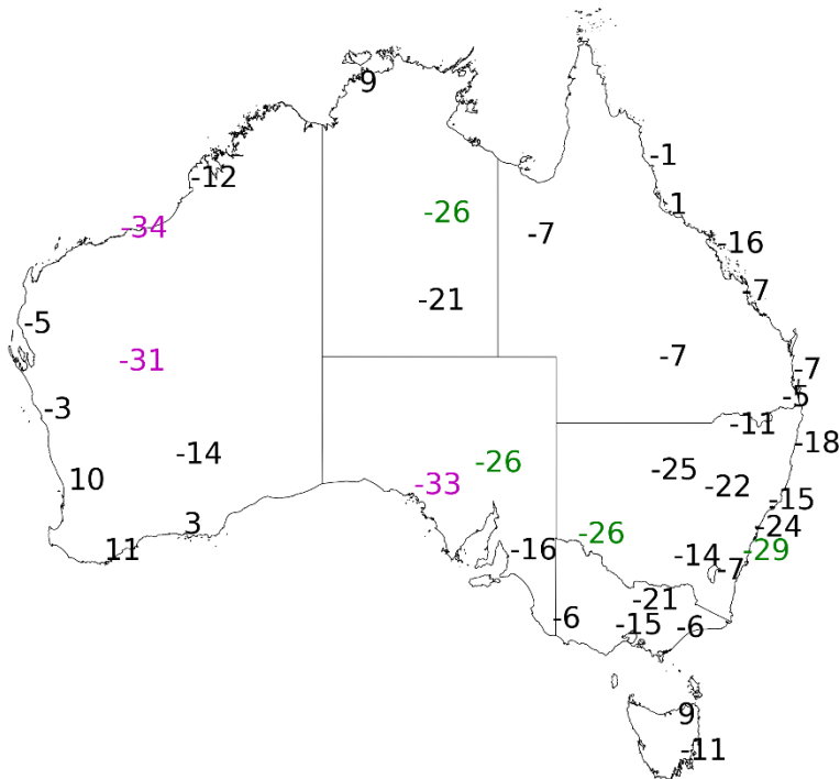
SON FFDI90-MAM SAM partial lag=2
